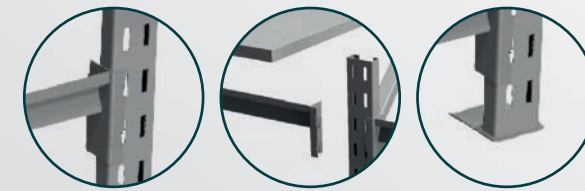
Longarinas de encaixe Longarinas com aba para reter a prateleira Laterais chumbadas no piso (opcional)
