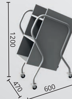
Ref: PSD1 painél senalizador duplo
